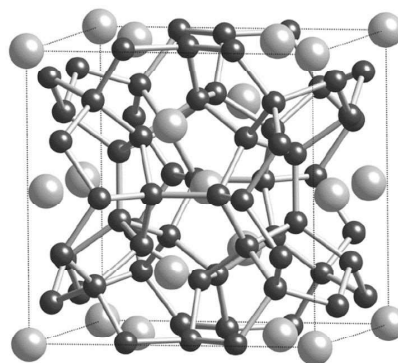
図2: カゴ状物質の単位構造
